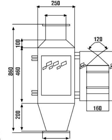
ME004-FTM FÜZE TİPİ MIKNATIS Missile Type Magnet مغناطيس اسطوانى
